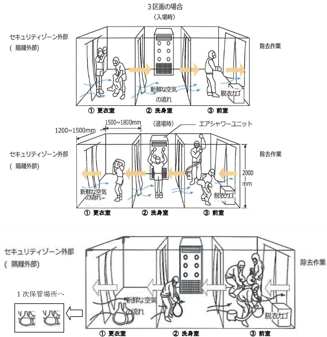
図-12 前室（セキュリティーゾーン）の例
