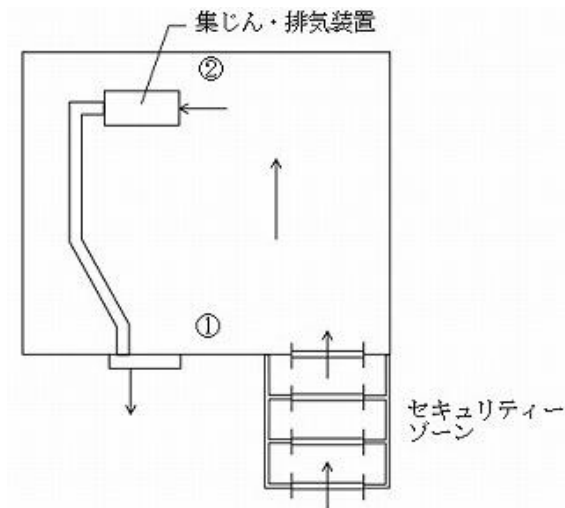
図-9 集じん・排気装置設置例
