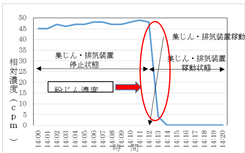
図 13-1 粉じん相対濃度計(デジタル粉じん計)による粉じん濃度減衰状況
