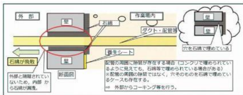
図－8 設備ダクト、配管等が壁を貫通している場合の注意事項
