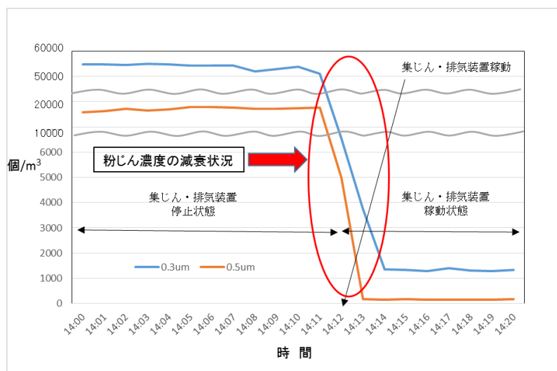
図 13-2 パーティクルカウンターによる粉じん濃度減衰状況
