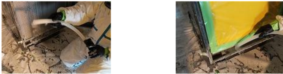
写真VI-12 スモークテスターによる確認
