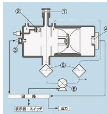
図-26 粉じん相対濃度計の構造の例
