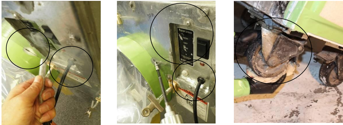
写真Ⅶ-3 漏れの発生しやすい箇所の例
