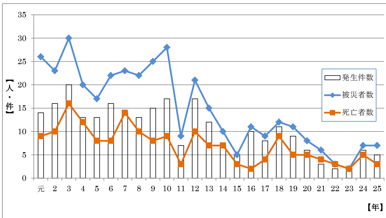
図2 硫化水素中毒の労働災害発生状況の推移（平成元年～平成25年）
